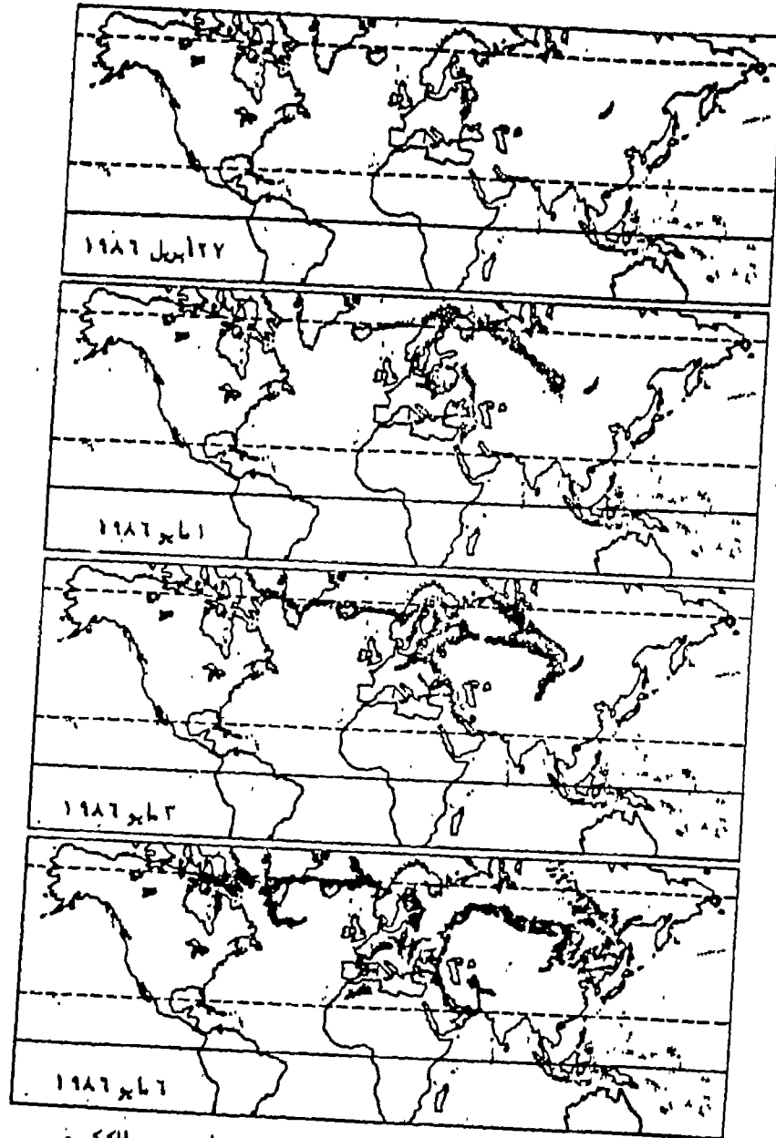
شكل (٥) : مسار السحابه الاشعاعيه لحادثه تشرنوبيل على مستوى الكوكب.
